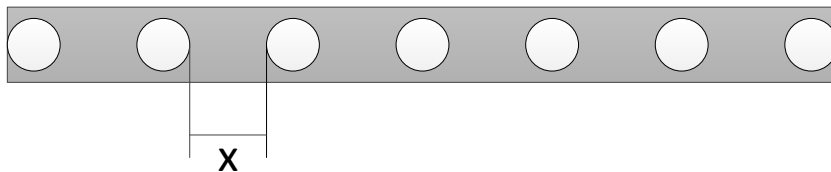
Abbildung 6-1: Schematische Darstellung einer NIR-Luftdüsenleiste mit einem Düsenabstand von 12,5 – 37,5 mm
